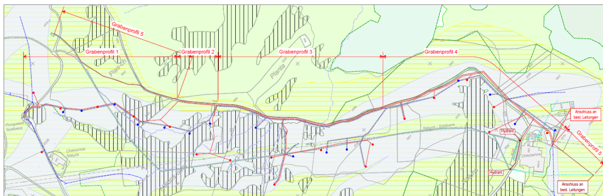
Condot da transport d'aua sü Schlivera / Motta Naluns
