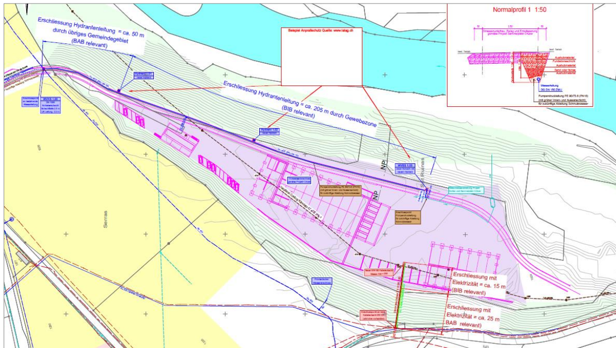
Areal da Sotruinas, Scuol
