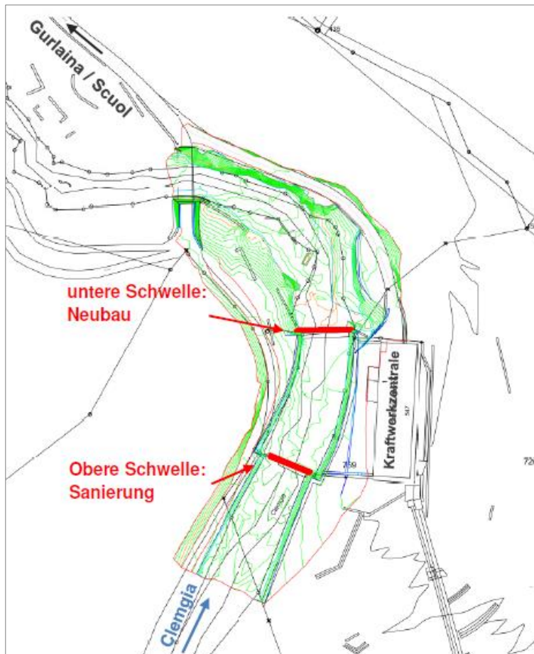
Scuol: Serras pro la centrala da l'ouvra electrica Clemgia
