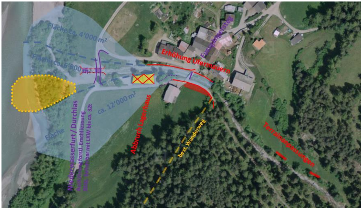
Illustraziun 2: Survista da las masüras previssas (cotschen = masüras construcziuns idraulicas; blau grischant = surfatschas da deposit potenzialas in cas da boudas; violet = concept d'access)
